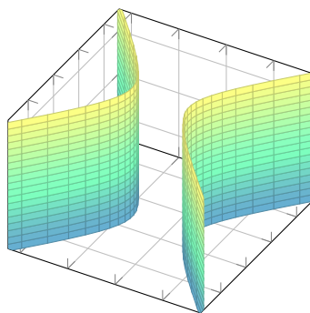
双曲柱面
