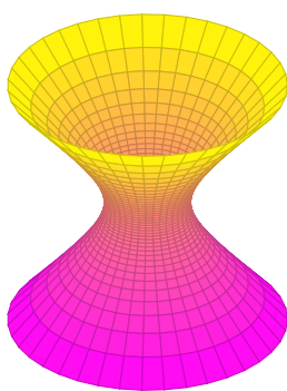
单叶双曲面
